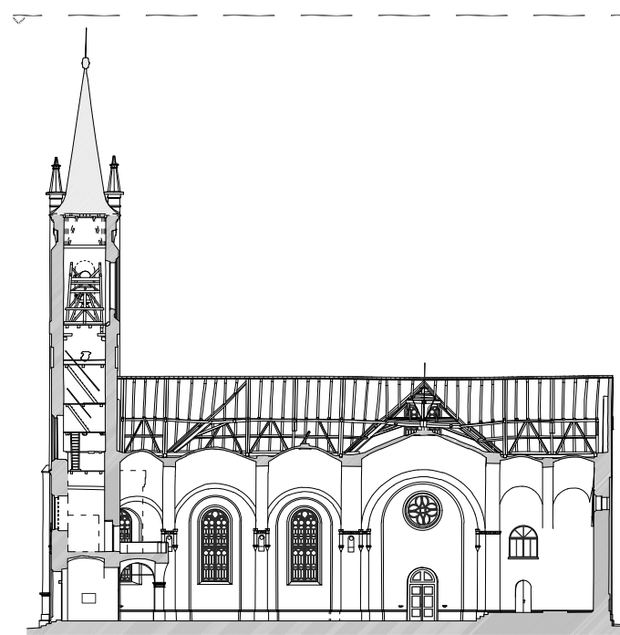
SHEMA: PRESJEK 1-1
